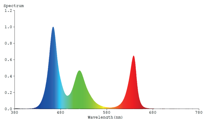
Spektrální graf MZ-RGB-1440-24V
